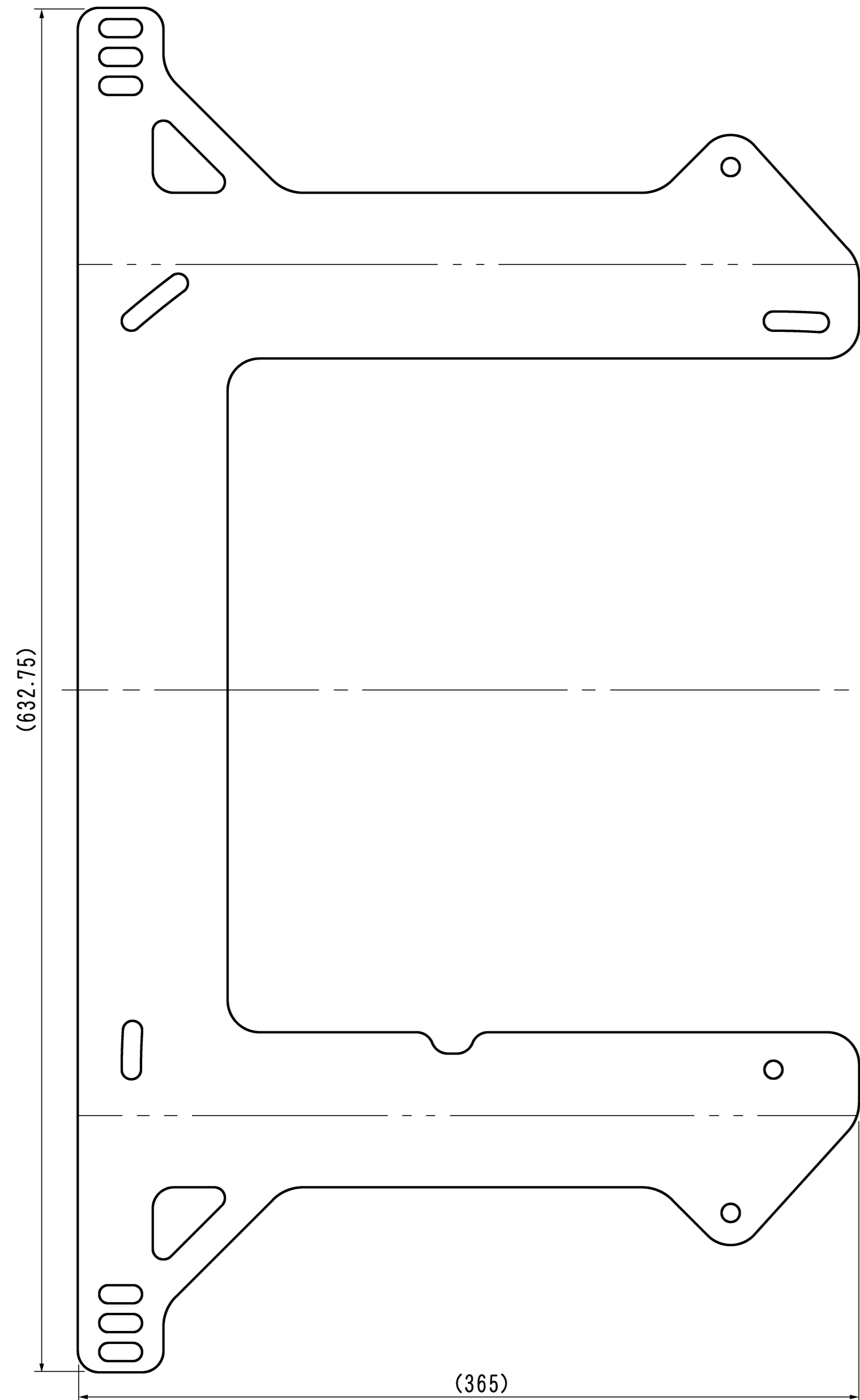
展開形状
